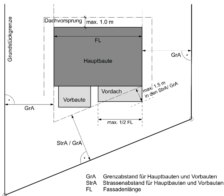
Abbildung 4: Grenz- und Strassenabstände von Vorbauten und Dachvorsprünge
