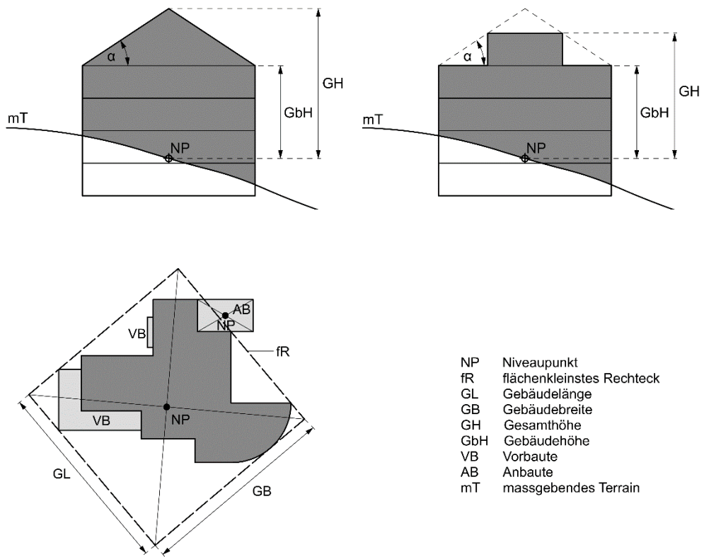
Abbildung 5: Niveaupunkt
