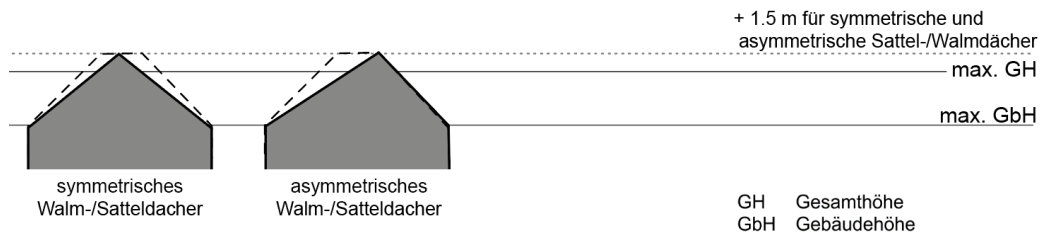
Abbildung 12: Mögliche Dachvarianten innerhalb Dachraumprofil - mit Zuschlag von 1.5 m
