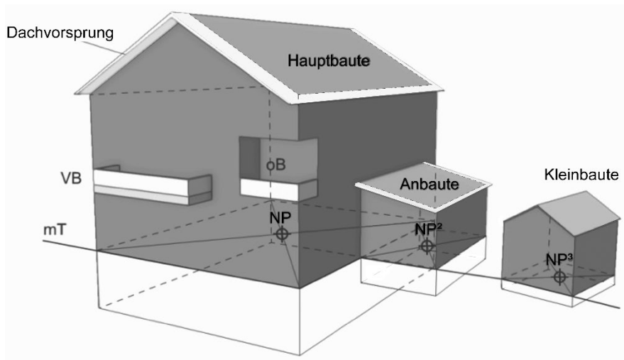
Abbildung 15: Berechnung Baumassenziffer
