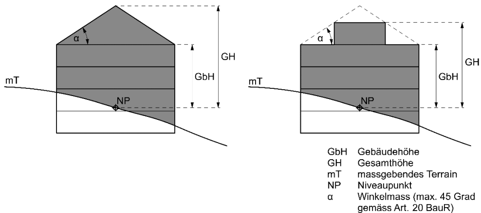
Abbildung 8: Gebäudehöhe, Gesamthöhe
