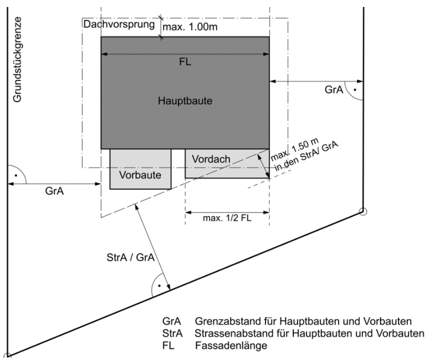
Abbildung 16: Grenzabstand
