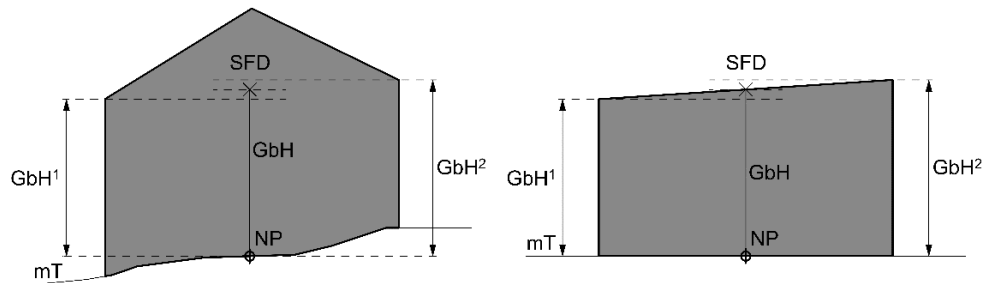
Abbildung 10: Ausgemittelter Schnittpunkt der Fassade mit der Dachoberkante
