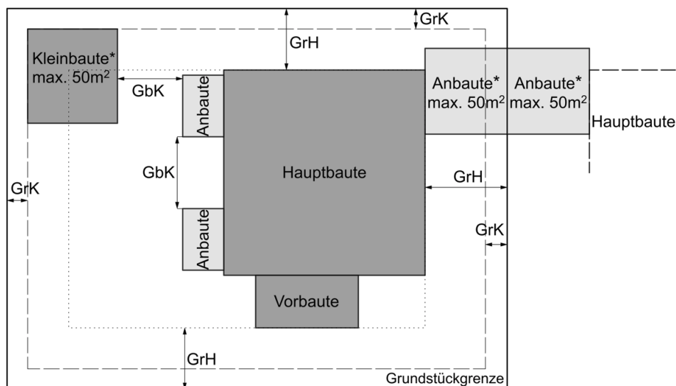
Abbildung 2: Kleinbauten und Anbauten
