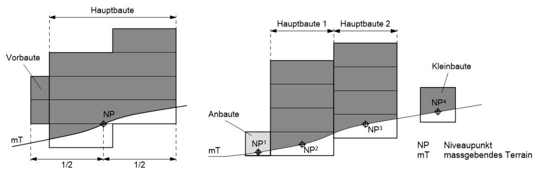
Abbildung 6: Separate Niveaupunkte
