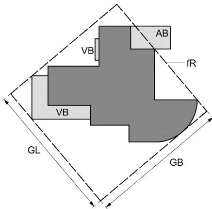
Abbildung 7: Flächenkleinstes Rechteck, Gebäudelänge, Gebäudebreite
