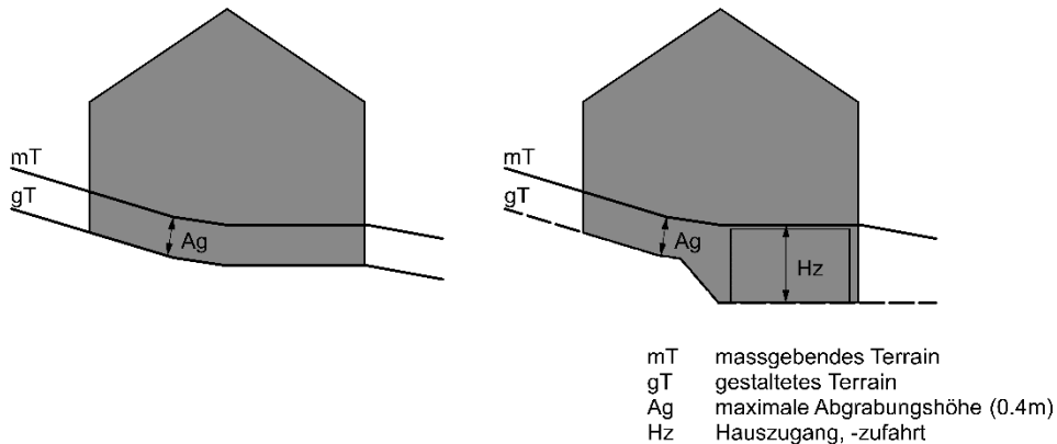
Abbildung 19: Maximale Abgrabungshöhe
