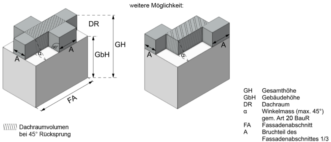
Abbildung 13: Flachdach
